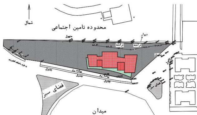
تصویر ۷. موقعیت و پلان ساختمان در دست احداث پژوهشکده که درون دانشگاه کردستان واقع شده است.
